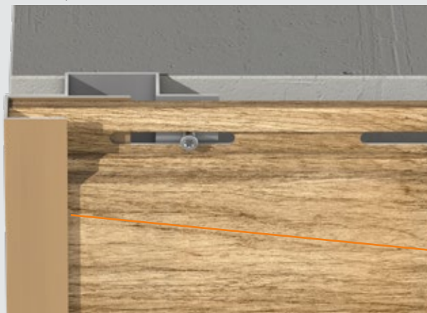
Abschluss-Startprofil
