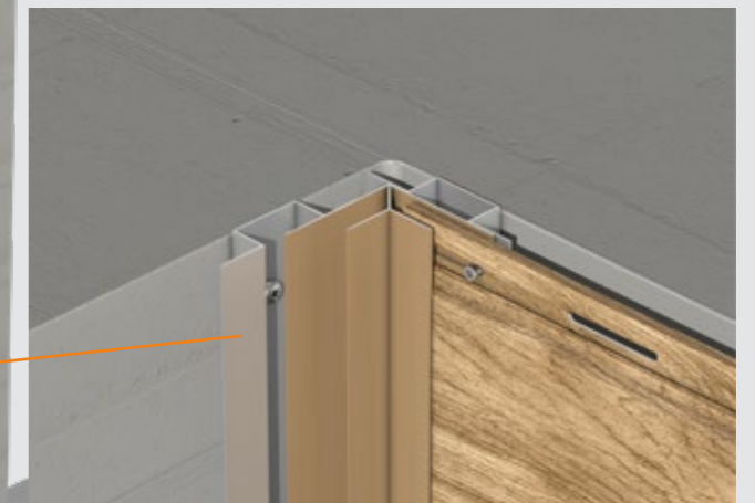
Innenecke
