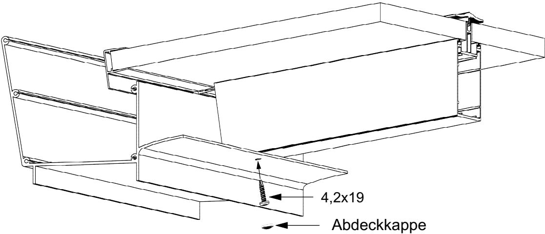
Detailskizze Montage Träger an Rinne
