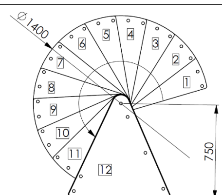
13 Stufen (Standard+1 Höhererweiterung) 13 steps (standard+1 height extension)
