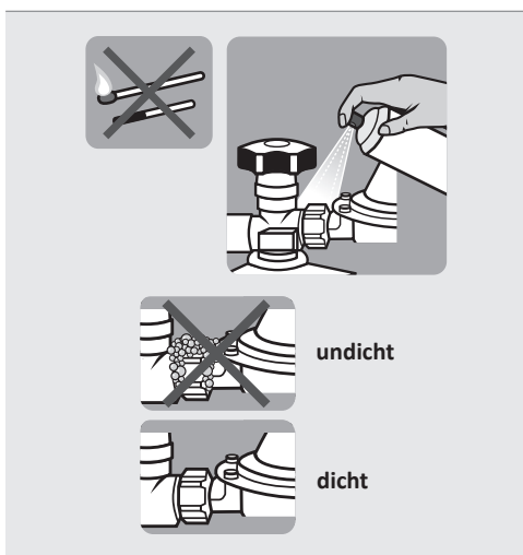
Abb.2: Dichtheitsprüfung
