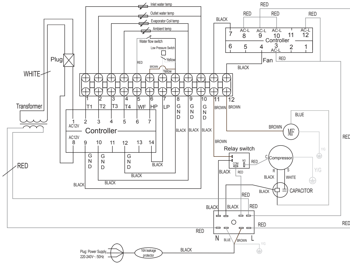
A.1 Wiring diagrams / Schaltpläne / Bedradingschema
