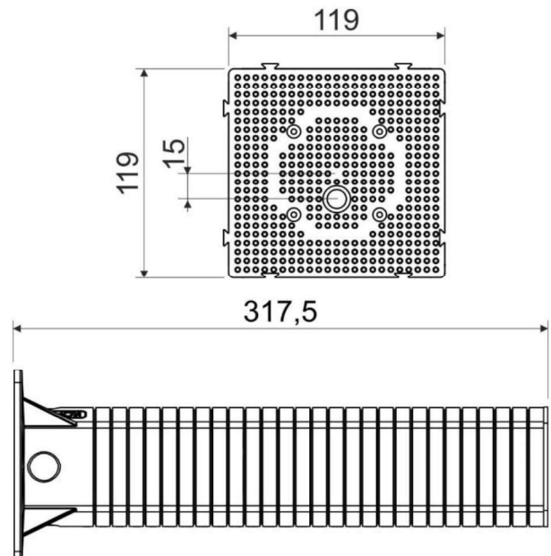
Montageplatte Wärmedämmung 300mm
