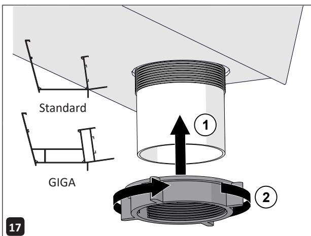
17 Drehen Sie die Verschraubung gegen den Uhrzeigersinn am Laubfänger fest. Achtung! Verleimen Sie den Laubfänger, wenn Sie eine GIGA-Rinne verwenden.
