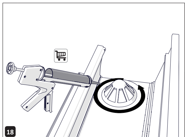
18 Verkitten Sie den Laubfänger.
