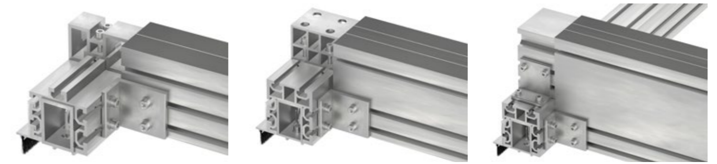
Alle Systemteile statisch geprüft mit FME Analyse und Statik Prüfbericht für Standard Rahmenabmessungen
