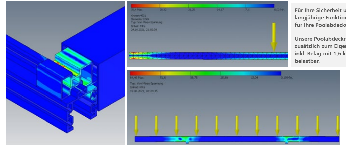
Alle Systemteile statisch geprüft mit FME Analyse und Statik Prüfbericht für Standard Rahmenabmessungen
